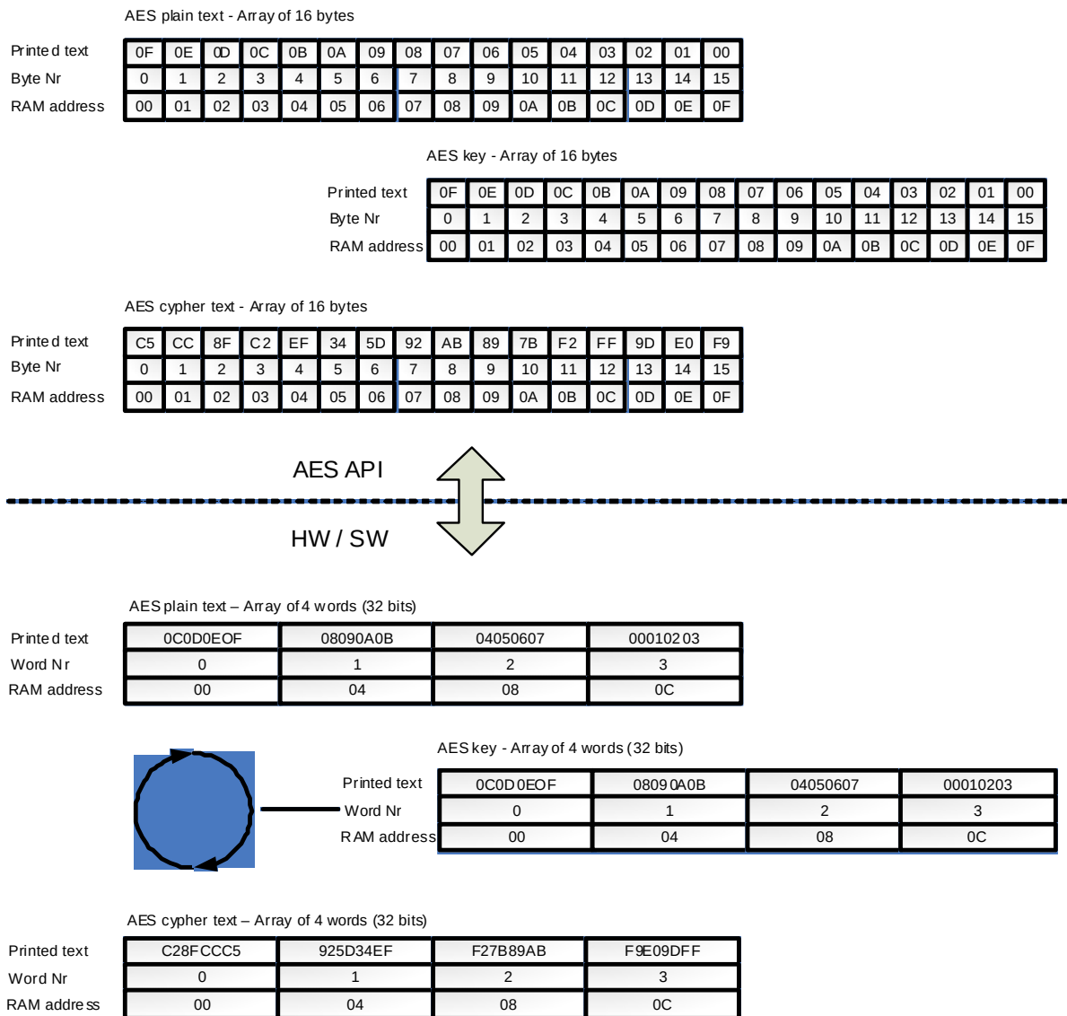
Fig 30. AES endianness
